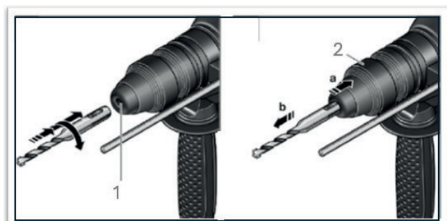
1 – Orifício de encaixe da broca (SDS Plus)
