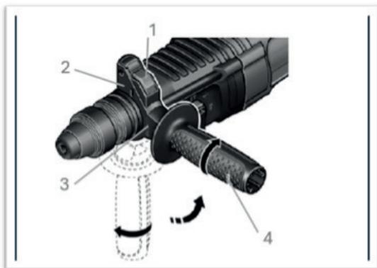
1 – Botão de travamento da barra de profundidade 2- anel de fixação 3- base da empunhadura 4- empunhadura lateral
